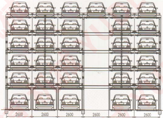
剖面图
